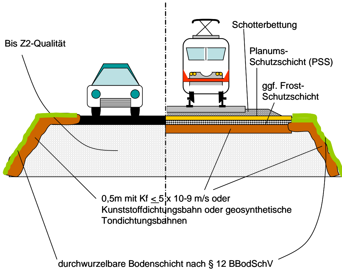
Abbildung 5-7 Regelbauweise Verkehrswegedamm
