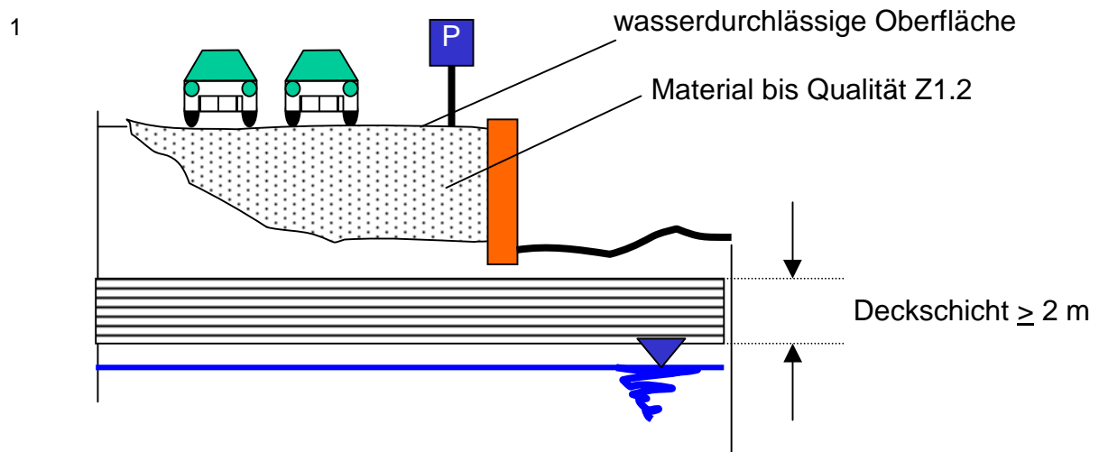
Abbildung 5-3: Z1.2 - Verwertung in technischen Bauwerken ohne definierte technische Sicherungsmaßnahmen, jedoch bei günstigen hydrogeologischen Verhältnissen
